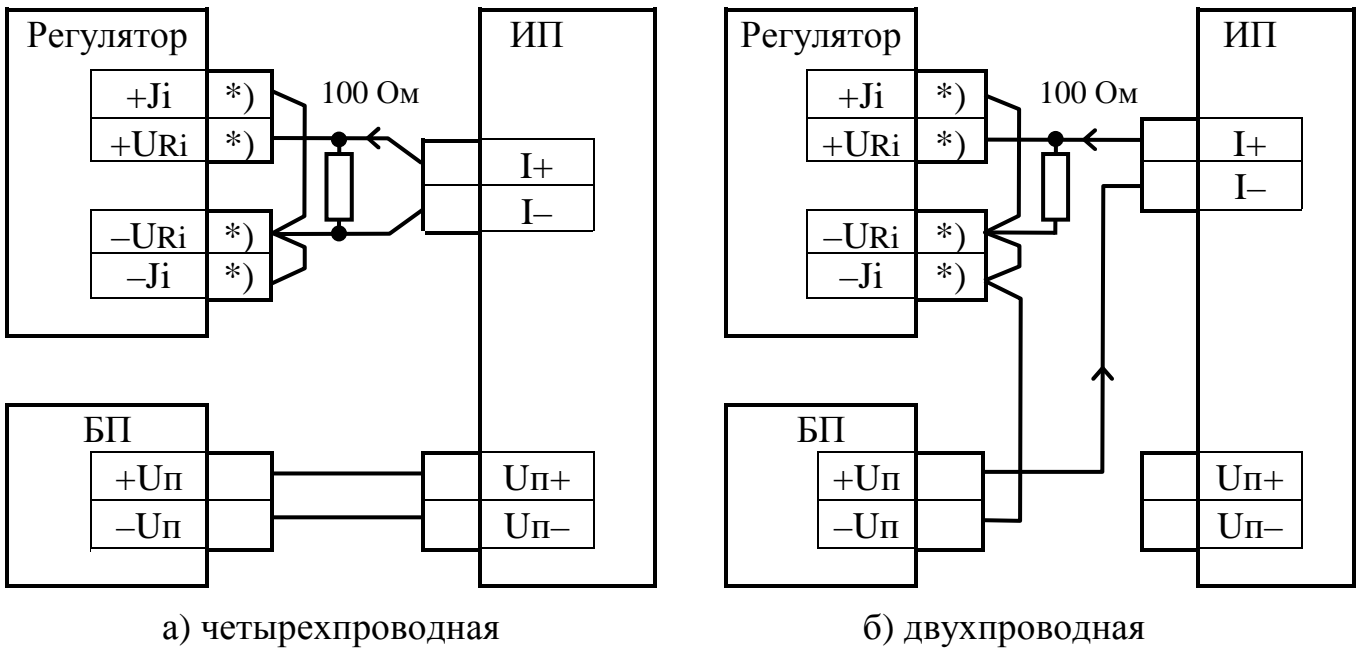
Рисунок 3.3 – Схемы подключения измерительных преобразователей с токовым выходом к регулятору исполнения 01
