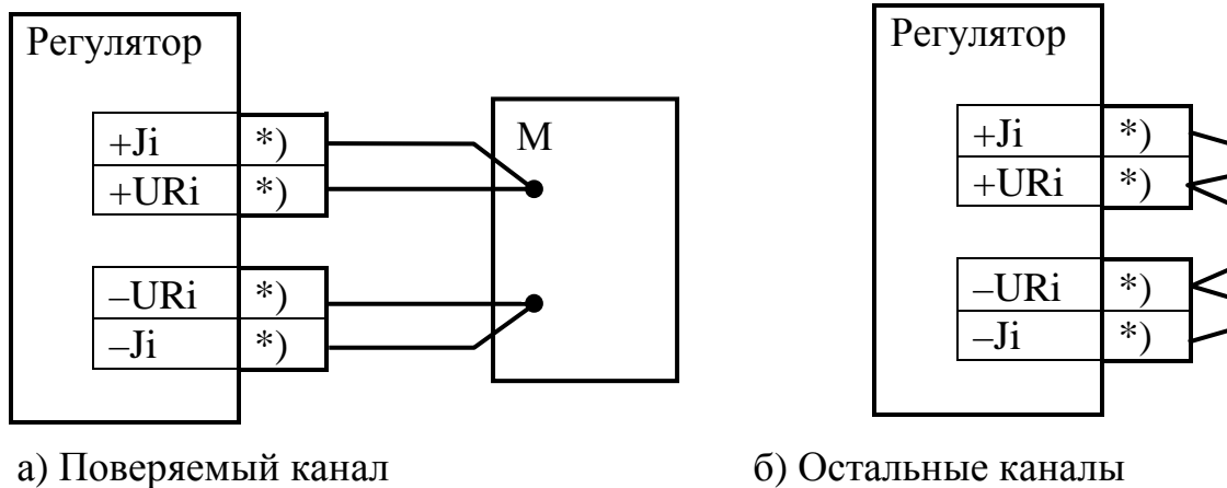
Рисунок 6.1 – Схема подключения средств поверки при проведении поверки ИК сопротивлений;
