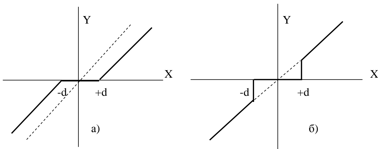
Рисунок 2.5 – зона нечувствительности
