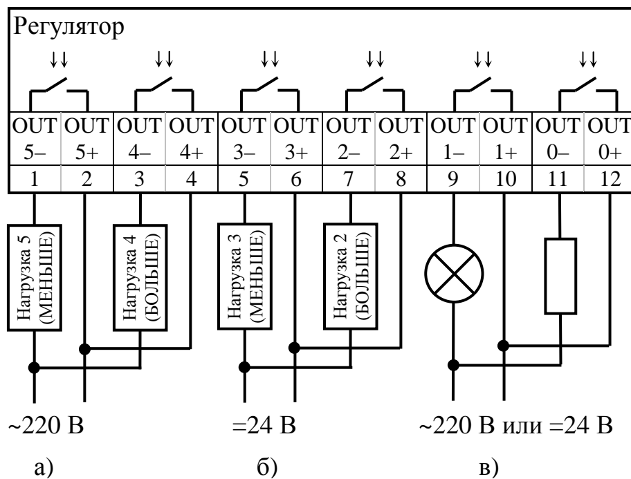
Рисунок 3.4 – Схема подключения нагрузок к выходам регулятора а) исполнительный механизм переменного тока; б) исполнительный механизм постоянного тока; в) другие исполнительные устройства, с работой по принципу «ВКЛ/ВЫКЛ» } работа по принципу «БОЛЬШЕ/МЕНЬШЕ»
