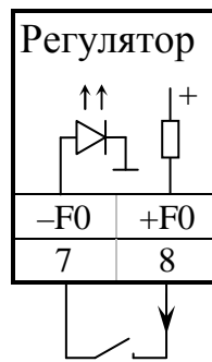
Рисунок 3.5 – Схема подключения датчика типа «сухой контакт» к дискретному входу регулятора (исполнение 01)
